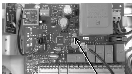
Knopf "RESET" bei KOMPACT / DOMO / KOMPACT PLUS (Box öffnen!)
