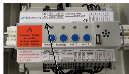
Knopf "RESET" bei CAFE/PREMIUM (Öffnen sie den Stromkasten!)
